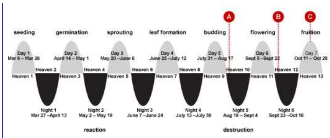
Abbildung 1. Die Kometen Honda und Elenin in Beziehung zu den Sieben Tagen und Sechs Nächten der Neunten Welle. A ist der kürzeste Abstand von Honda zur Erde. B zeigt die Zeit des Durchgangs von Elenin zwischen der Sonne und der Erde und C ist seine kürzeste Distanz zur Erde.
